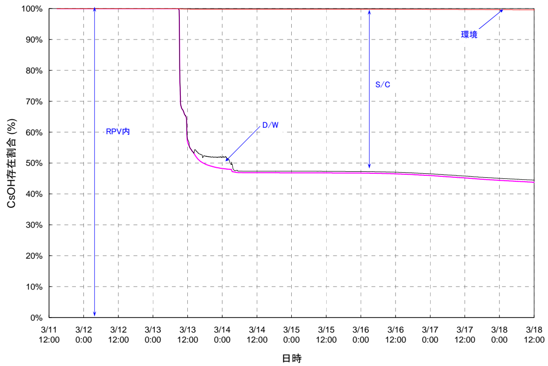
図 3. 3. 2. 8 3号機 FP の存在割合 (2 / 2) 【その2】
