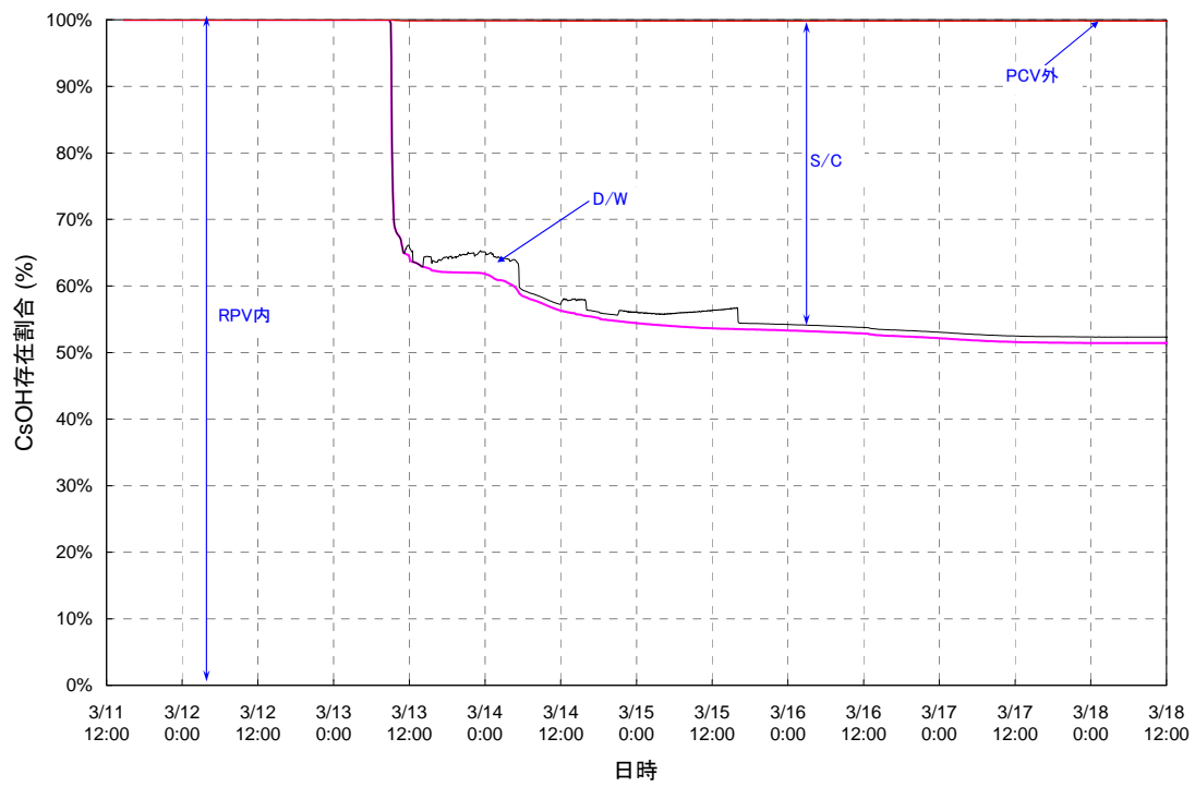
図 3. 3. 1. 8 3号機 FP の存在割合 (2 / 2) 【その 1】
