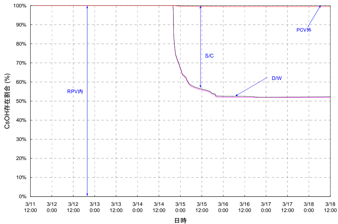
図 3. 2. 2. 8 2号機 FPの存在割合 (2 / 2) 【その2】
