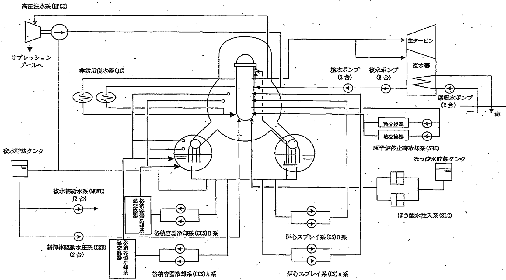
図-1. 1 福島第一原子力発電所1号炉の設備構成の概要
