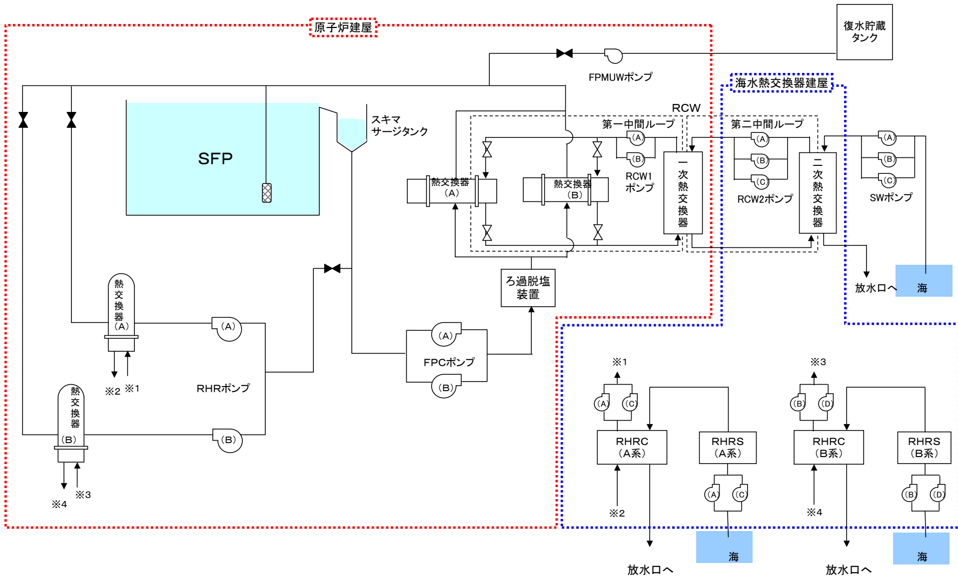
1号機 FPC系統概略図
