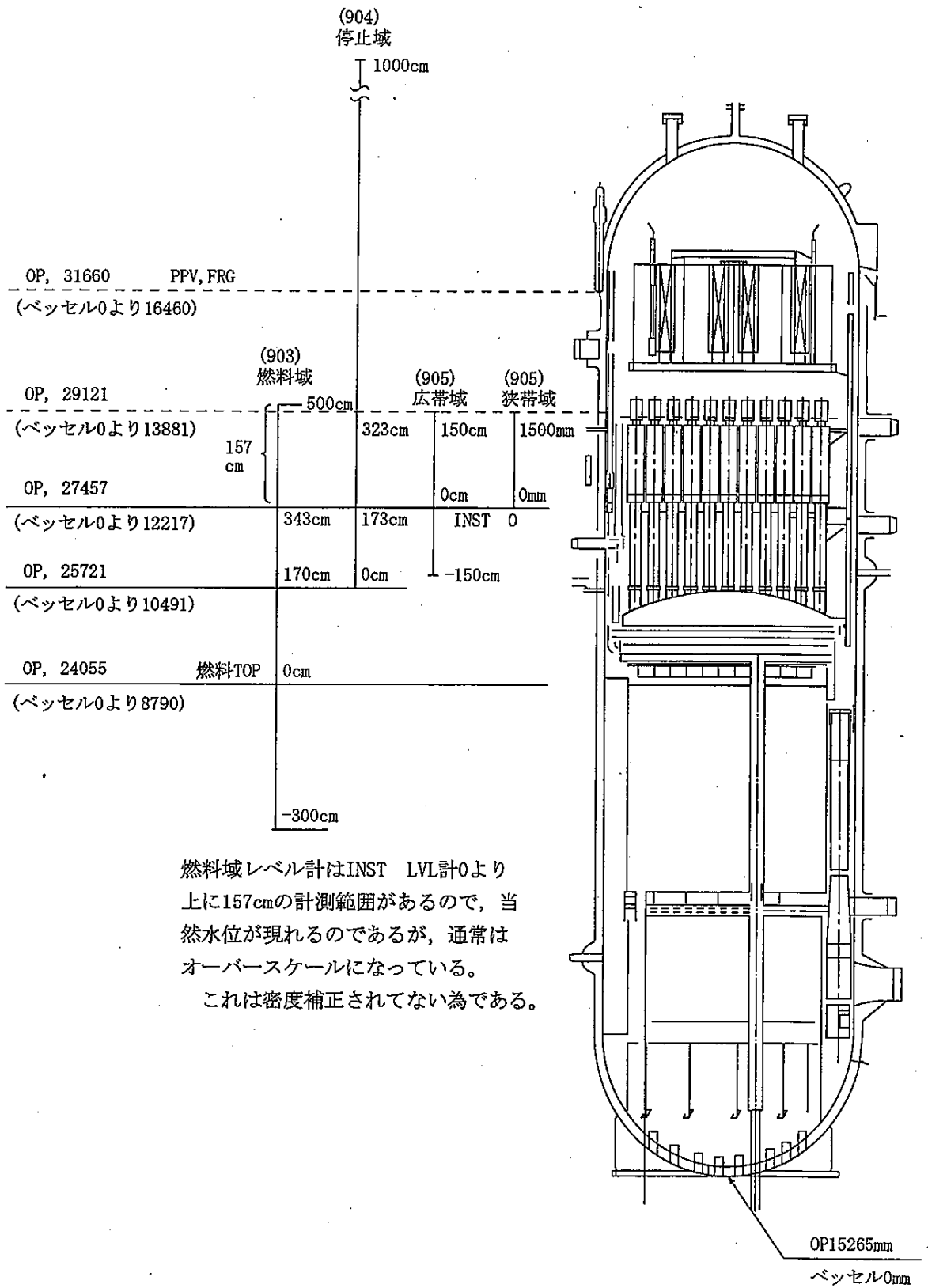
図1 原子炉水位計の指示範囲
