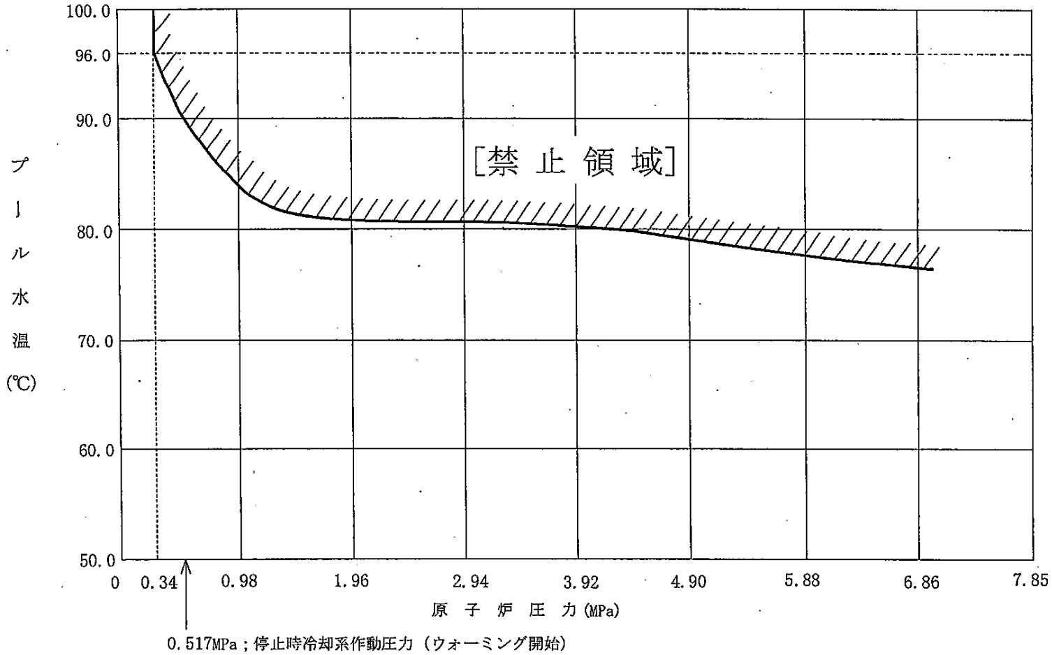
図C-2 S / P熱容量制限値
