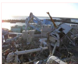
RHRポンプ
