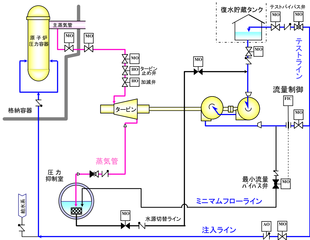
図1 HPCI 系統概略図
