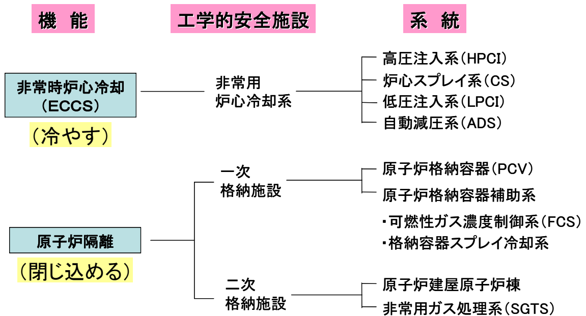
工学的安全施設の構成（BWR - 4 の例）
